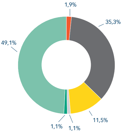
Verbleibende Energieträgermix
