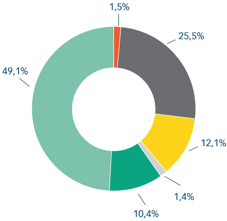
Energieträgermix Deutschland
